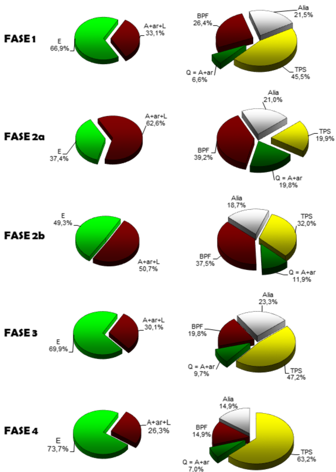
Fig. 2 – Ex Cava a Filo: evoluzione del paesaggio vegetale e dell’ambiente. Valori pollinici medi dei singoli raggruppamenti per fasi: Legnose (A+ar+L); Erbacee (E); TPS = Praterie Steppiche Freddi; Q (A+ar) = Querceto; BPF = Bosco Pleistocenico Freddo; Alia .
