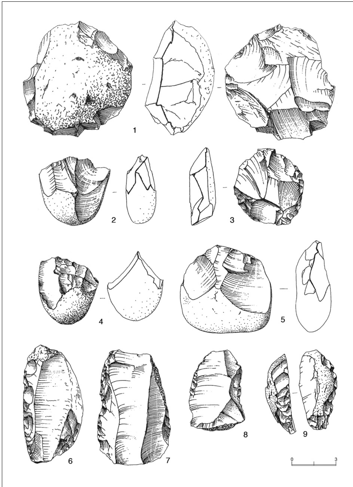
Fig. 1 – San Lazzaro di Savena (BO), Cave I.E.C.M.E. (Inghiottittoi A e B). 1, 3: nuclei; 2, 4-5: chopping-tools ; 6-8: raschiatoi; 9: raschiatoio denticolato (disegni G. Almerigogna).
