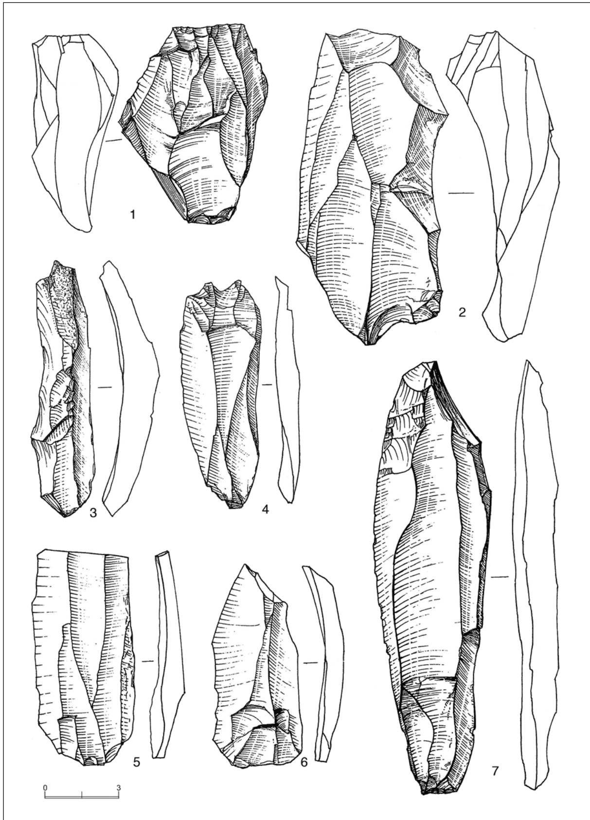
Fig. 3 – San Lazzaro di Savena (BO), Cave I.E.C.M.E. (Inghiottoio S.I.A.). 1: nucleo sub-piramidale; 2: scheggia laminare sorpassata; 3: lama a cresta; 4-7: lame (disegni A. M. Monaco).
