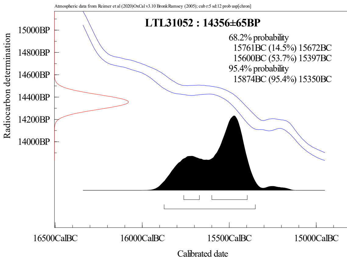
Figura 1. Calibrazione della data convenzionale al radiocarbonio del campione LTL31052
