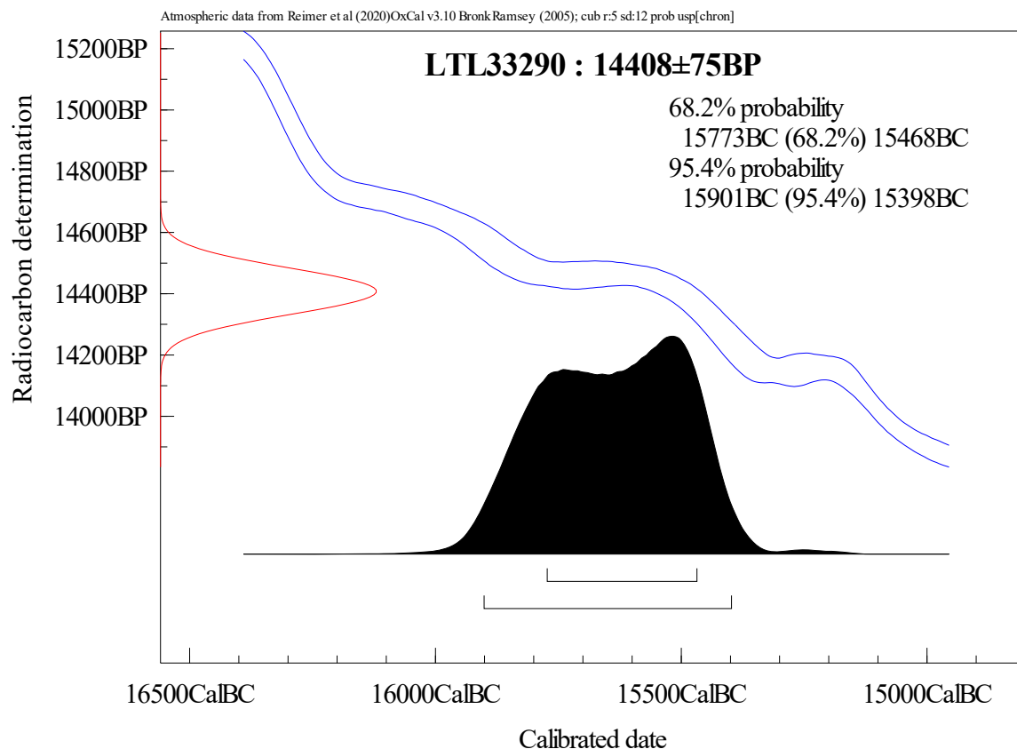
Figura 1. Calibrazione della data convenzionale al radiocarbonio del campione LTL33290
