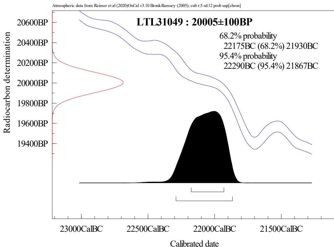
Figura 1. Calibrazione della data convenzionale al radiocarbonio del campione LTL31049
