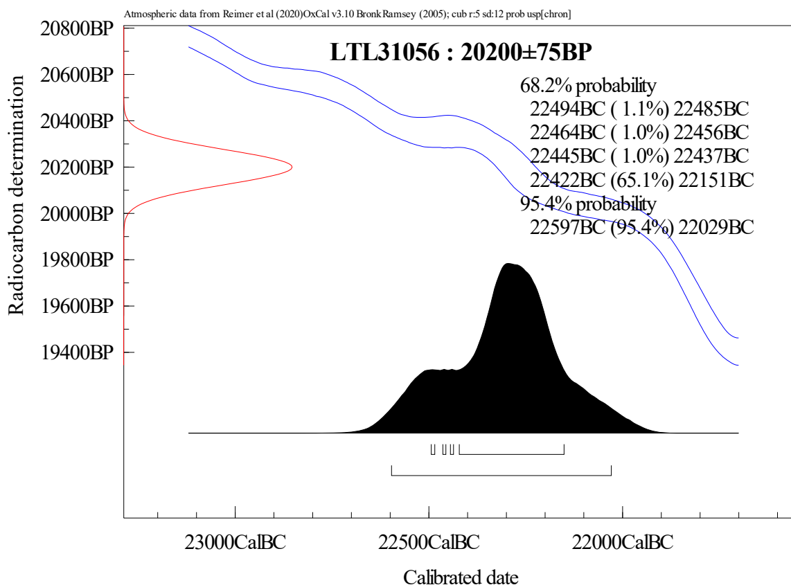
Figura 1. Calibrazione della data convenzionale al radiocarbonio del campione LTL31056
