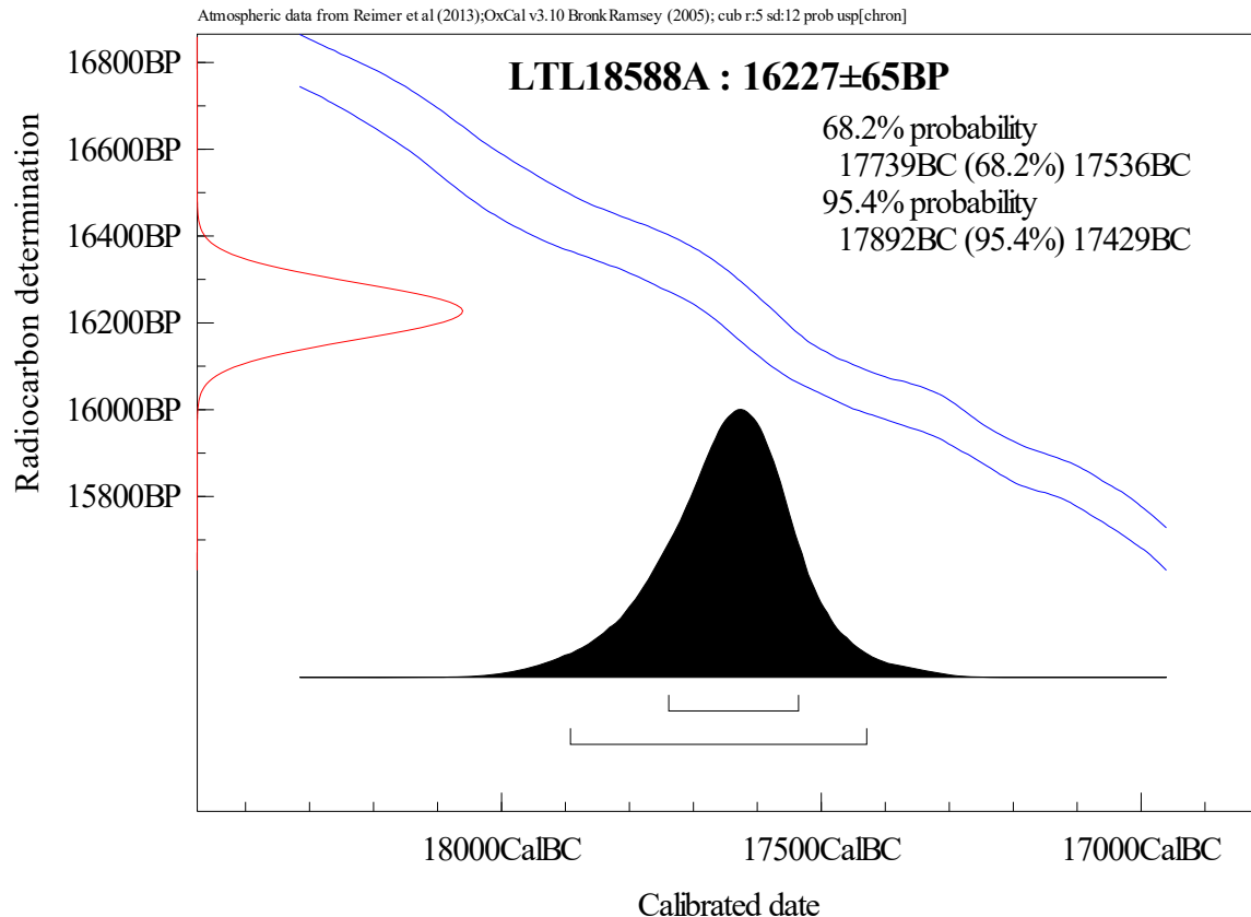
Figura 1. Calibrazione della data convenzionale al radiocarbonio del campione LTL18588A
